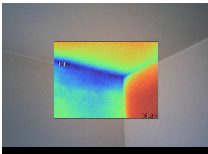
Korter 9 Külmasild lae ja seina liitekohas.
