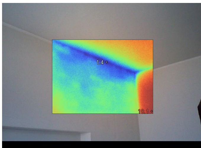
Korter 9 Külmasild lae ja seina liitekohas.
